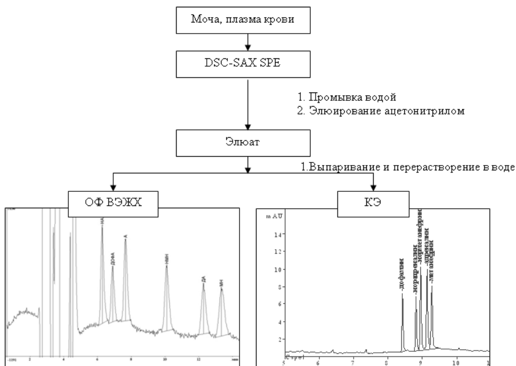
Рис. 3. Схема твердофазной экстракции катехоламинов, ДОФА и метанефринов из биологической жидкости с использованием патрона DSC-SCX
