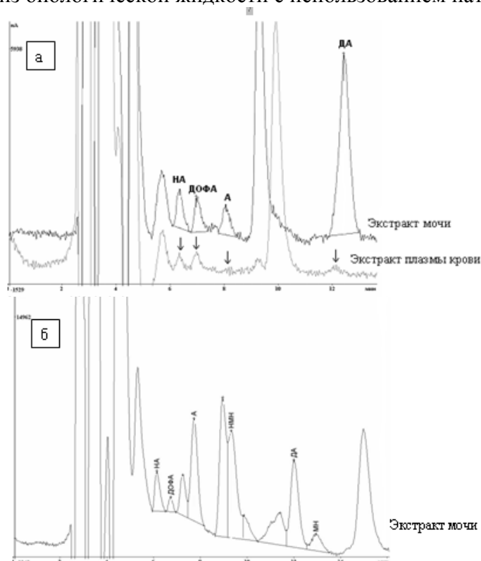
Рис. 4. Хроматограмма экстракта мочи и плазмы крови при различных вариантах ТФЭ: (а) сорбент Al_2O_3 , (б) картридж DSC-SCX. Прибор: Waters 590 с амперометрическим детектированием, напряжение на рабочем электроде +0,85 В), колонка Ascentic C18 (5 мкм, 4,6 x 250 мм). Скорость потока подвижной фазы 1 мл/мин, объем пробы 100 мкл.
