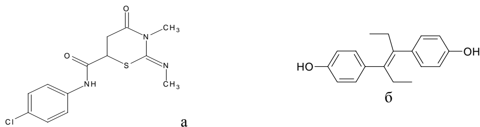
Рис. 1. Структура молекул 4-хлоранилида 5,6-дигидро-2-метилимино-3-метил-1,3-тиазин-4-он-6-карбоновой кислоты (а) и транс -4,4'-дигидрокси- \alpha,\alpha' -диэтилстильбена (б).
