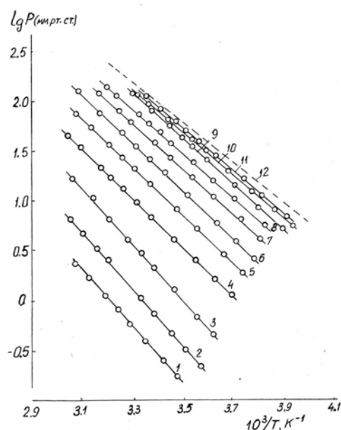
Рис.2. Изостеры адсорбции паров метилового спирта на тетраметиламмониевом монтмориллоните, соответствующие различным количествам адсорбированного вещества (моль/кг): 1-1.24, 2-1.50, 3-1.82, 4-2.19, 5-2.50, 6-2.81, 7-3.14, 8-3.46, 9-4.05, 10-4.50, 11-4.91, 12 - зависимость \text{Lg}P_s от T^{-1} для неадсорбированного метилового спирта
