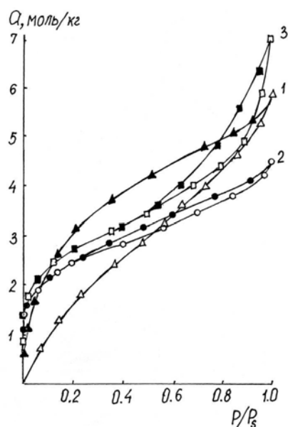
Рис. 1. Изотермы адсорбции паров метилового спирта при 293К на натриевом (1), метиламмониевом (2) и тетраметиламмониевом (3) монтмориллонитах
