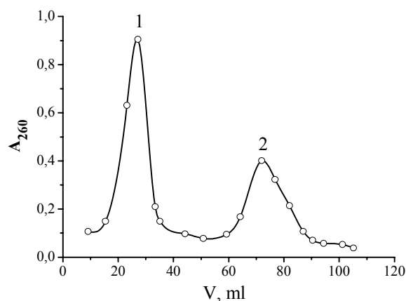
Рис. 2. Гельхроматограмма исходного раствора тимусаминна (рН 10,2); (1) – высокомолекулярная фракция, содержащая ДНК, (2) – низкомолекулярная фракция, содержащая олигонуклеотиды и пептиды. Колонка 1,6 x 32 см, Сефадекс G-50 (superfine), элюент 0.05M NaCl
