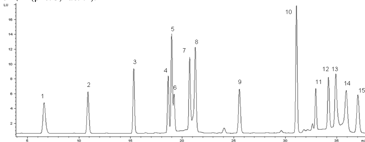
Рис. 3. Хроматограмма смеси ОФА/НМЦ производных аминокислот. Колонка «Zorbax Eclipse AAA» (4.6x150 мм) с предколонкой. Градиентное элюирование. Скорость потока 1 мл/мин. T = 30^{\circ}\text{C} . Детектор – флуориметрический ( \lambda_{\text{возб.}}=340 \text{ нм} , \lambda_{\text{регистр.}}=450 \text{ нм} ). Градиентное элюирование: 0 мин, 10%A, 90%B; 5 мин, 10%A, 90%B; 18 мин, 24%A, 76%B; 22 мин, 24%A, 76%B; 30 мин, 40%A, 60%B; 35 мин, 40%A, 60%B; 37 мин, 90%A, 10%B; 47 мин, 90%A, 10%B, 50 мин 10%A, 90%B, 57 мин 10%A, 90%B, где А-метанол/ацетонитрил/вода (225мл/225мл/5мл), В-0.01 М \text{Na}_2\text{HPO}_4 , pH 6.0. 1=Asp, 2=Glu, 3=Ser, 4=Thr, 5=Gly, 6=His, 7=Arg, 8=Ala, 9=Tyr, 10=Val+ Met, 11=Trp, 12=Phe, 13=Ile, 14=реагент+ Leu, 15=Lys.
