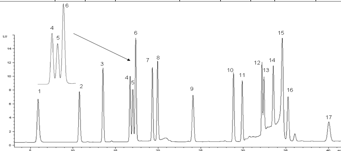
Рис. 4. Хроматограмма смеси ОФА/ИБЛЦ производных аминокислот.
