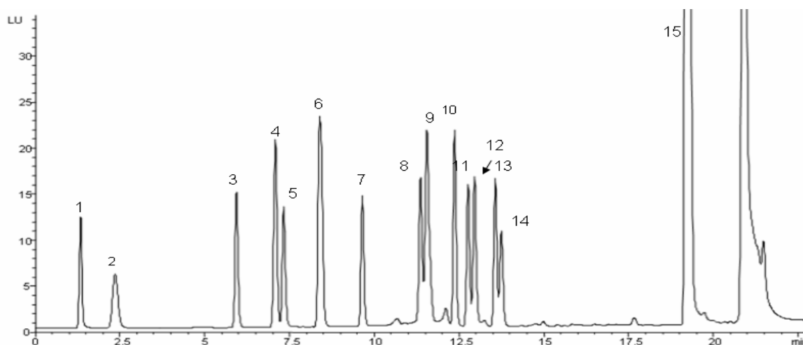
Рис. 2. Хроматограмма смеси ОФА/3-МРА производных аминокислот после анализа 60 проб. Колонка «Zorbax Eclipse AAA» (4.6x150 мм) с предколонкой.
