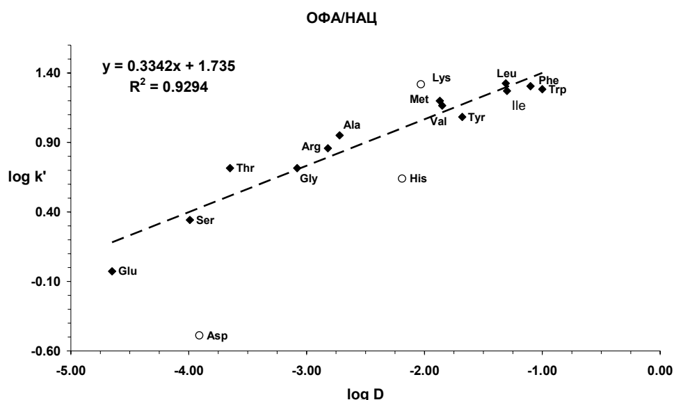
Рис. 5. Зависимость логарифма фактора удерживания от логарифма коэффициента распределения для производных аминокислот с ОФА/НАЦ
