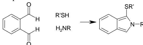
Рис. 1. Схема реакции аминокислоты с o -фталевым альдегидом.
