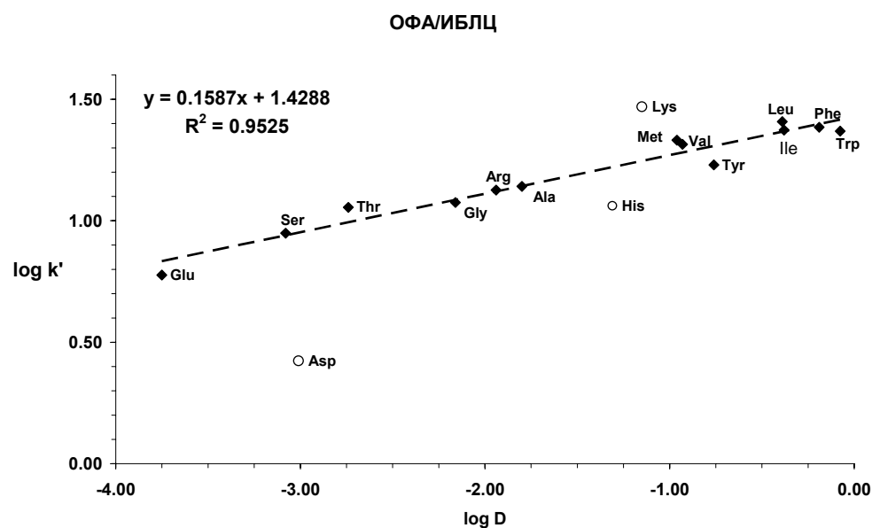
Рис. 7. Зависимость логарифма фактора удерживания от логарифма коэффициента распределения для производных аминокислот с ОФА/ИБЛЦ
