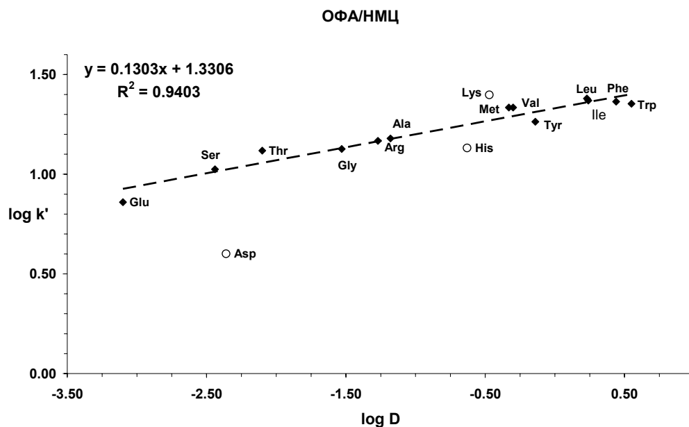
Рис. 6. Зависимость логарифма фактора удерживания от логарифма коэффициента распределения для производных аминокислот с ОФА/НМЦ
