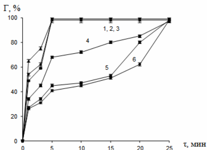
Рис. 4. Зависимость степени извлечения 1-(4сульфофенил)-3-метил-5-(бензоксазол-2-ил)формазанатов Cu(II) (1), Co(II) (2), Ni(II) (3), Cd(II) (4), Zn(II) (5), Pb(II) (6) при их совместном присутствии из раствора от времени контакта фаз
