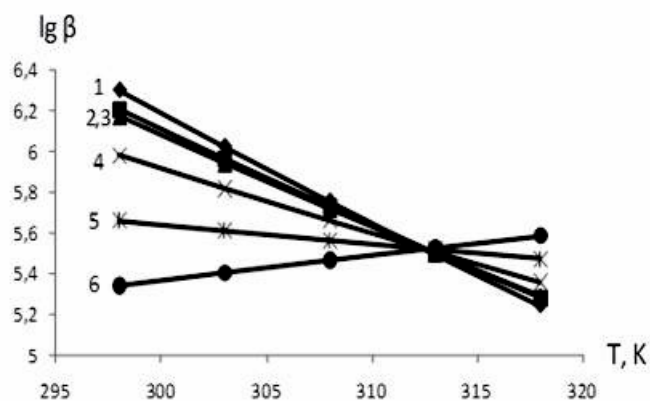
Рис. 2. Зависимость констант стабильности от температуры и ионной силы комплексов ионов \text{Fe}^{2+} с диизопропилдитиофосфатом натрия: [\text{NaNO}_3] = 0 (1); 0.075 (2); 0.1 (3); 0.25 (4); 0.5 (5) и 0.75 М (6)
