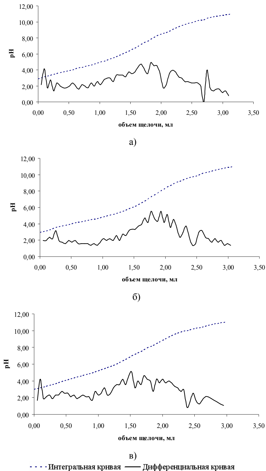
Рис. 1. Результаты прямого потенциометрического титрования комплексов ГК-ТМ а) холостое титрование без соли ТМ; б) кадмий; в) медь
