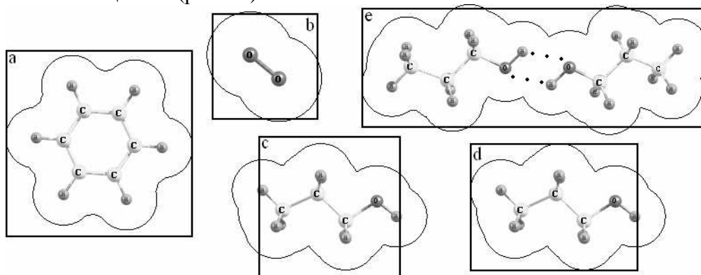
Рис. 2. Сопоставление размеров молекул бензола (а), кислорода (b) и n -пропанола (с–е) с учётом ван-дер-ваальсовых радиусов с размерами молекулярных площадок
