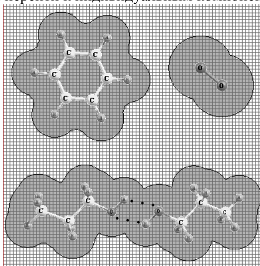
Рис. 3. Молекулярные площадки кислорода, бензола и n -пропанола, представленные совокупностью ячеек
