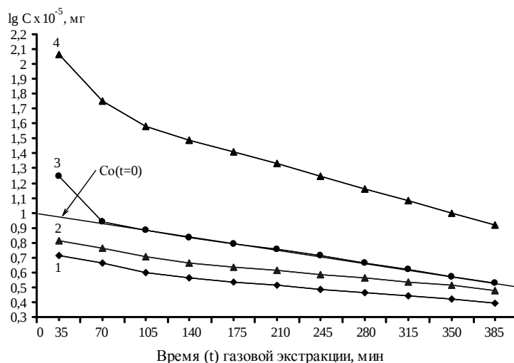
Рис. 1. Зависимость логарифма концентрации акрилонитрила и диметилформамида, выделяющихся из ПАН-волокна при температуре 100 °С, от время газовой экстракции: 1 – акрилонитрил из ПАН-волокна марки С, 2 – акрилонитрил из ПАН-волокна марки Д, 3 – акрилонитрил из ПАН-волокна марки С, содержащий сажу, 4 – диметилформамид из ПАН-волокна марки Д. Вес образца 0.15 г. Камера из стекла объёмом 1.3 см 3 . Экстрагировали 60 см 3 азота органические вещества из ПАН-волокна, концентрировали на ПФХ и вводили из патрона-концентратора в аналитическую колонку методом термической десорбции
