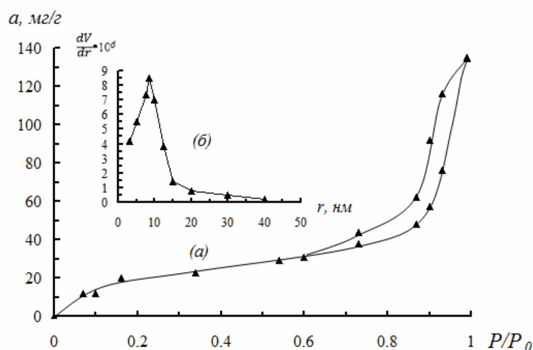
Рис. 1. Изотерма адсорбции паров воды на Н-форме глины (а) и распределение пор по радиусам (б)
