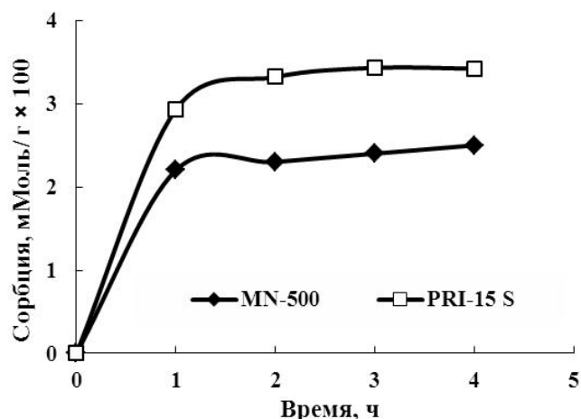
Рис. 1. Кинетика сорбции фосфатов на MN-500/Fe и PRI-15S/Fe в мМоль на грамм сырого сорбента; 1 мМоль фосфатный буфер pH 7.5, соотношение v/m = 50:1 (мл/г сырого полимера)
