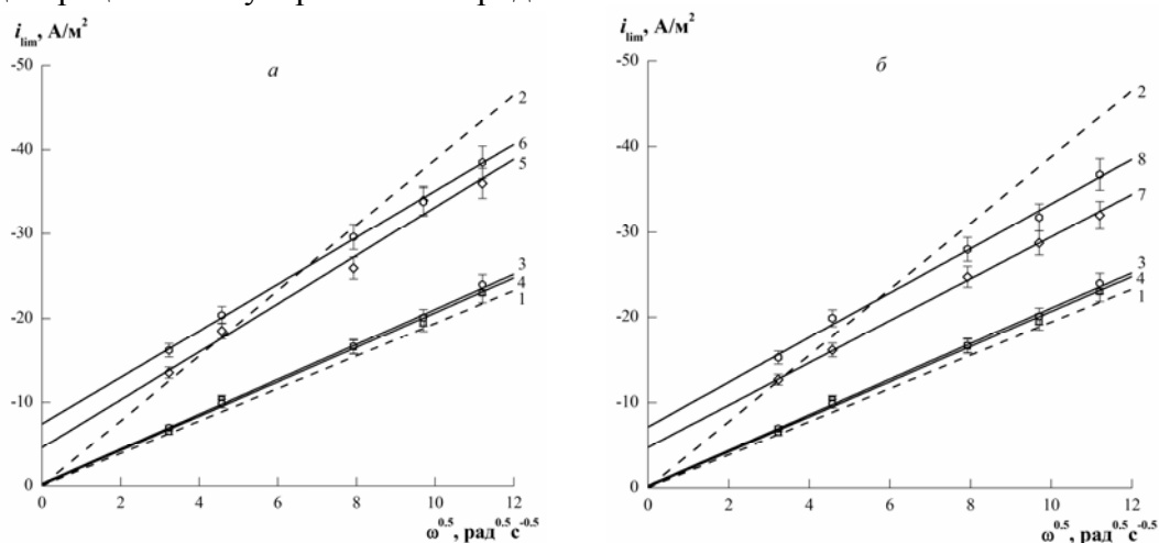
Рис. 5. Зависимость предельной плотности тока i_{lim} электровосстановления кислорода от корня квадратного из скорости вращения электрода \omega для систем: 1 – теоретический двухэлектронный механизм; 2 – теоретический четырехэлектронный механизм; 3 – компактный графитовый электрод; 4 – МФ-4СК/АУ; 5 – Ag/МФ-4СК/АУ, восстановитель N_2H_4 ; 6 – Ag/МФ-4СК/АУ, восстановитель – NaBH_4 ; 7 – Cu/МФ-4СК/АУ, восстановитель – N_2H_4 ; 8 – Cu/МФ-4СК/АУ, восстановитель – NaBH_4 .
