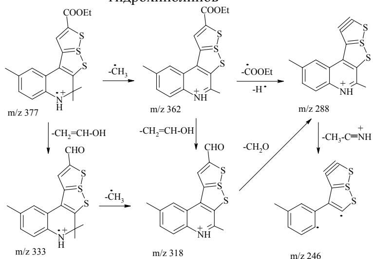
Схема 2. Фрагментация молекулярного иона 2(3)-карбэтокси-5,9,9-триметил-8,9-дигидрохино[3,4-в]-1,6,6а( \lambda^4 )-триапенталена
