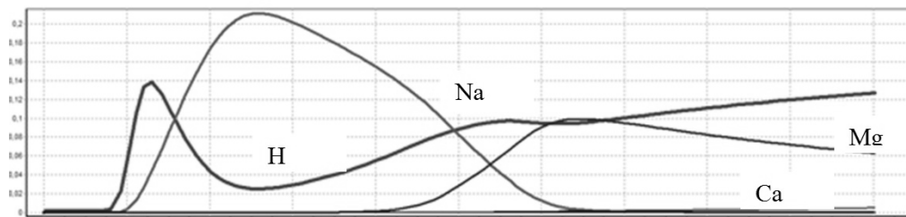
Рис. 7. Выходные кривые регенерации катионита КУ-2 0.179M H 2 SO 4
