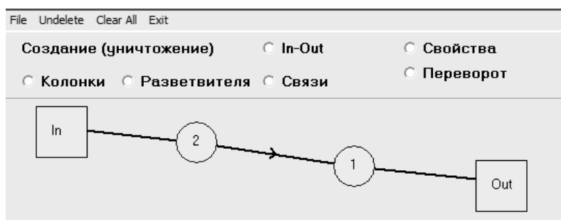
Рис. 5. Схема ступенчатого противотока
