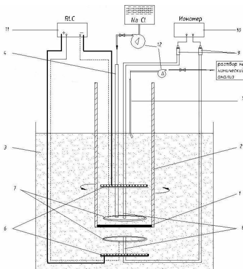
Рис. 1. Электрическая и гидродинамическая схема установки с ВМД: 1 – мембрана; 2 – вращающаяся верхняя полуячейка с раствором; 3 – нижняя полуячейка с раствором; 4 и 5 – капилляры для подвода и отвода раствора; 6 – Pt поляризующие электроды; 7 – Pt измерительные зонды (кольца); 8 – капилляры Лuggина-Габера; 9 – электроды сравнения Ag/AgCl; 10 – иономер; 11 – измеритель-анализатор переходных характеристик и импеданса
