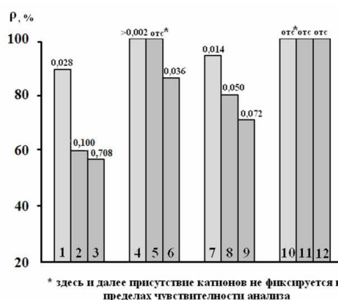
Рис. 1. Влияние концентрации гидрокарбоната натрия ( C_{соли} ), продолжительности ( \tau_c ) и числа стадий сорбции на глубину извлечения ( \rho ) катионов Ca(II) из 0.25 М раствора CaCl_2 . C_{соли} , мг/дм 3 : 1, 4, 7 и 10 – отсутствует; 2, 5, 8 и 11-84; 3, 6, 9 и 12-840; \tau_c , мин.: 1...6-20; 7...12-40. Число последовательных стадий сорбции 1...3 и 7...9-1; 4...6 и 10...12-2.
