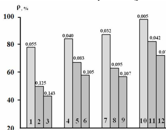
Рис. 2. Влияние концентрации гидрокарбоната натрия ( C_{\text{соли}} ), продолжительности ( \tau_c ) и числа стадий сорбции на глубину извлечения ( \rho ) катионов \text{Mg(II)} из 0.25 \text{ М} раствора \text{MgCl}_2 . C_{\text{соли}}, \text{ мг/дм}^3 : 1, 4, 7 и 10 – отсутствует; 2, 5, 8 и 11-84; 3, 6, 9 и 12 – 840; \tau_c, \text{ мин.} : 1...6-20; 7...12-40. Число последовательных стадий сорбции 1..3 и 7...9-1; 4...6 и 10...12-2
