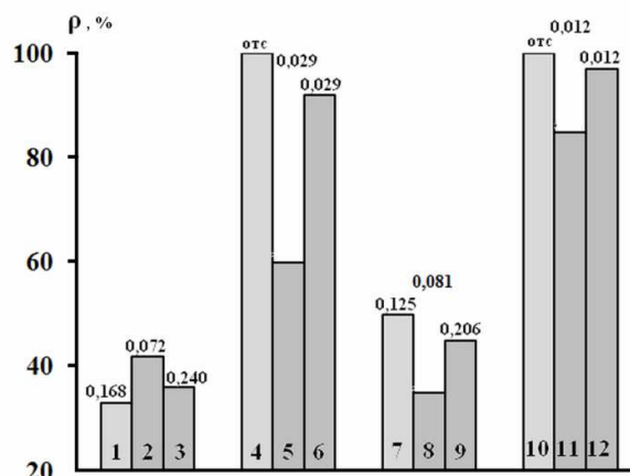
Рис. 5. Влияние продолжительности ( \tau_c ) и числа стадий на глубину сорбции катионов \text{Ca}^{2+} (1, 4, 7 и 10), \text{Mg}^{2+} (2, 5, 8 и 11) и \text{Ca}^{2+} и \text{Mg}^{2+} совместно (3, 6, 9 и 12) концентратом глауконита из раствора, содержащего 0.25 \text{ M CaCl}_2 + 0.125 \text{ M MgCl}_2 + 10^{-2} \text{ M NaHCO}_3 . Масса сорбента – 1 \text{ г}/0.1 \text{ дм}^3 раствора
