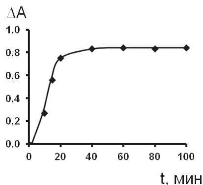
Рис. 5. Зависимость оптической плотности плёнок, модифицированных ПГК, от времени выдерживания в растворе белка (сукцинатный буфер с pH 2.5; C_{Mo(VI)}=4.0 \cdot 10^{-5} M , C_{\text{белка}} 0.1 \text{ г/л} ; \lambda=600 \text{ нм} ; C_{\text{ПГК исх.}}=1.0 \cdot 10^{-3} M )
